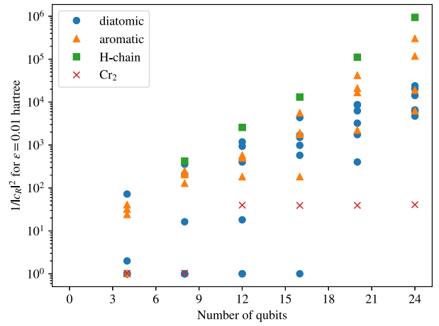
(d) 1/|c_R|^2 for energy error \epsilon = 0.01 Hartree.
